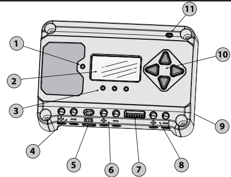
Abbildung 2.1 – EcoPulse Ausstattung
