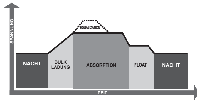
Abbildung 4.1 – EcoPulse Ladealgorithmus
