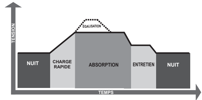
Figure 4.1. Algorithme de charge de l'EcoPulse
